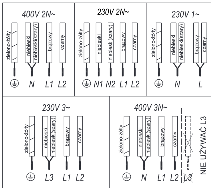
Rys. 6a (5 PRZEWODÓW)
