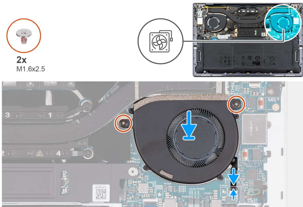
Rysunek 31. Instalowanie lewego wentylatora
