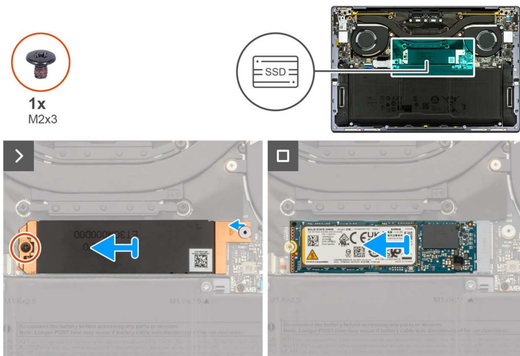
Rysunek 27. Wymontowywanie dysku SSD M.2 2280
