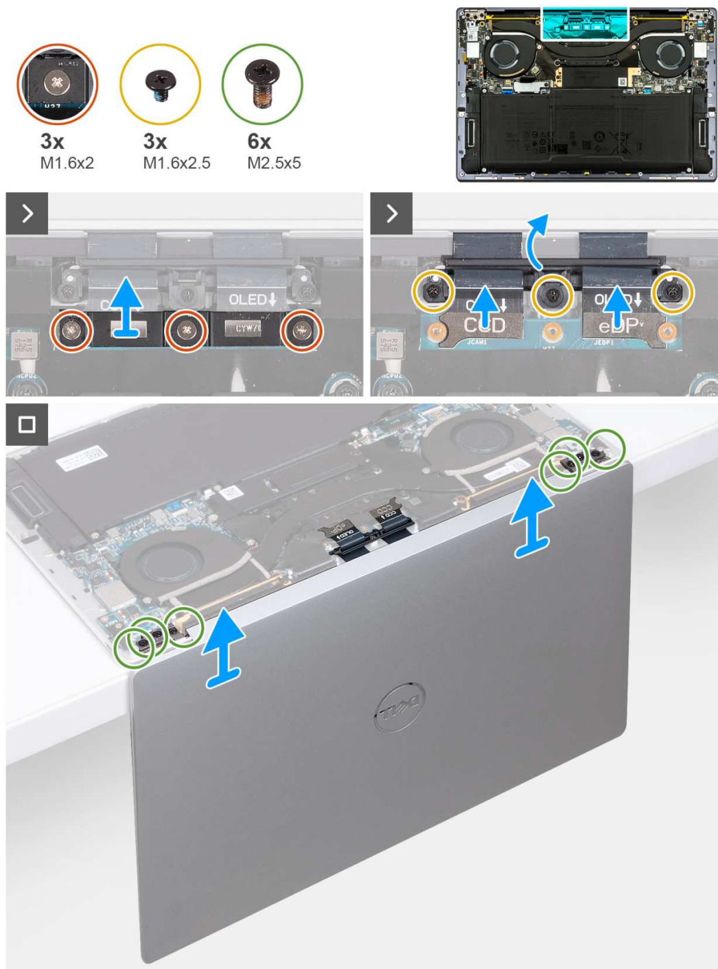
Rysunek 35. Wymontowywanie zestawu wyświetlacza
