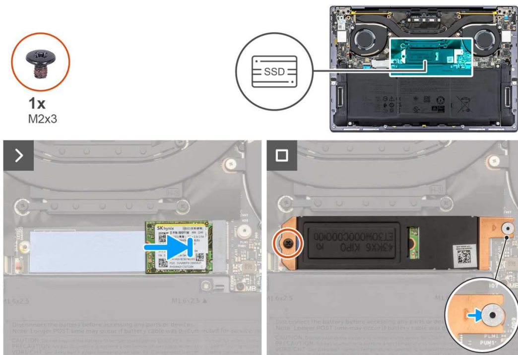
Rysunek 26. Instalowanie dysku SSD M.2 2230
