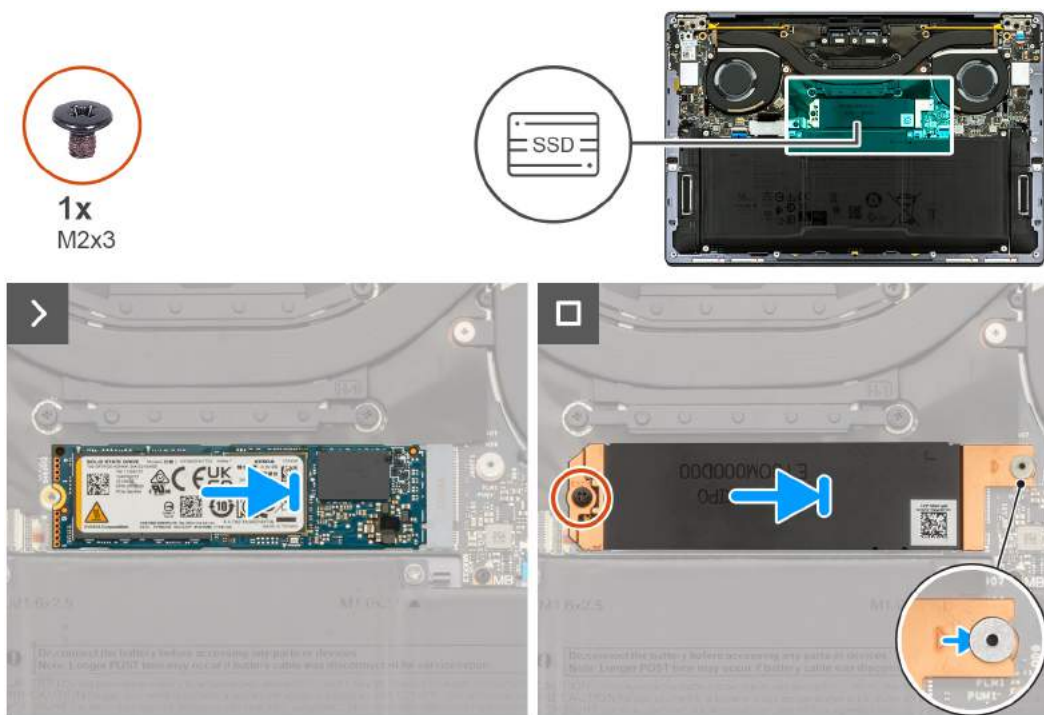
Rysunek 28. Instalowanie dysku SSD M.2 2280
