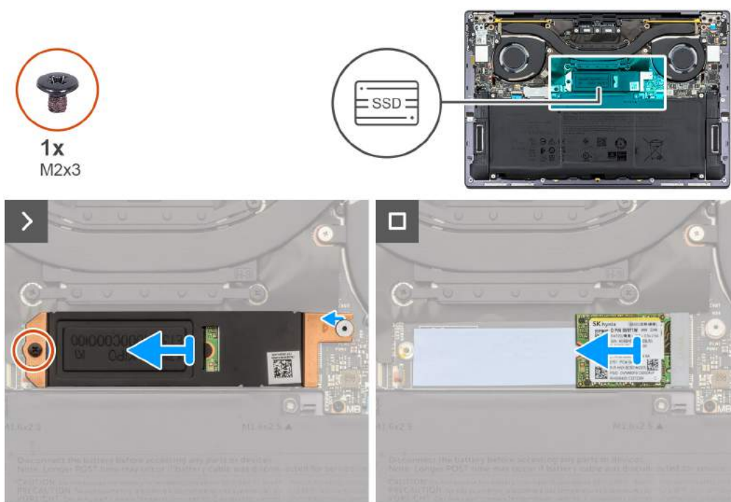
Rysunek 25. Wymontowywanie dysku SSD M.2 2230
