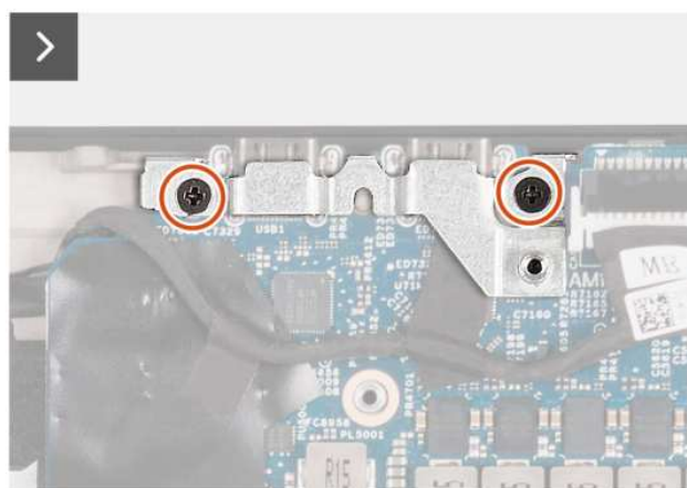
Rysunek 39. Wymontowywanie klamry złącza Type-C
