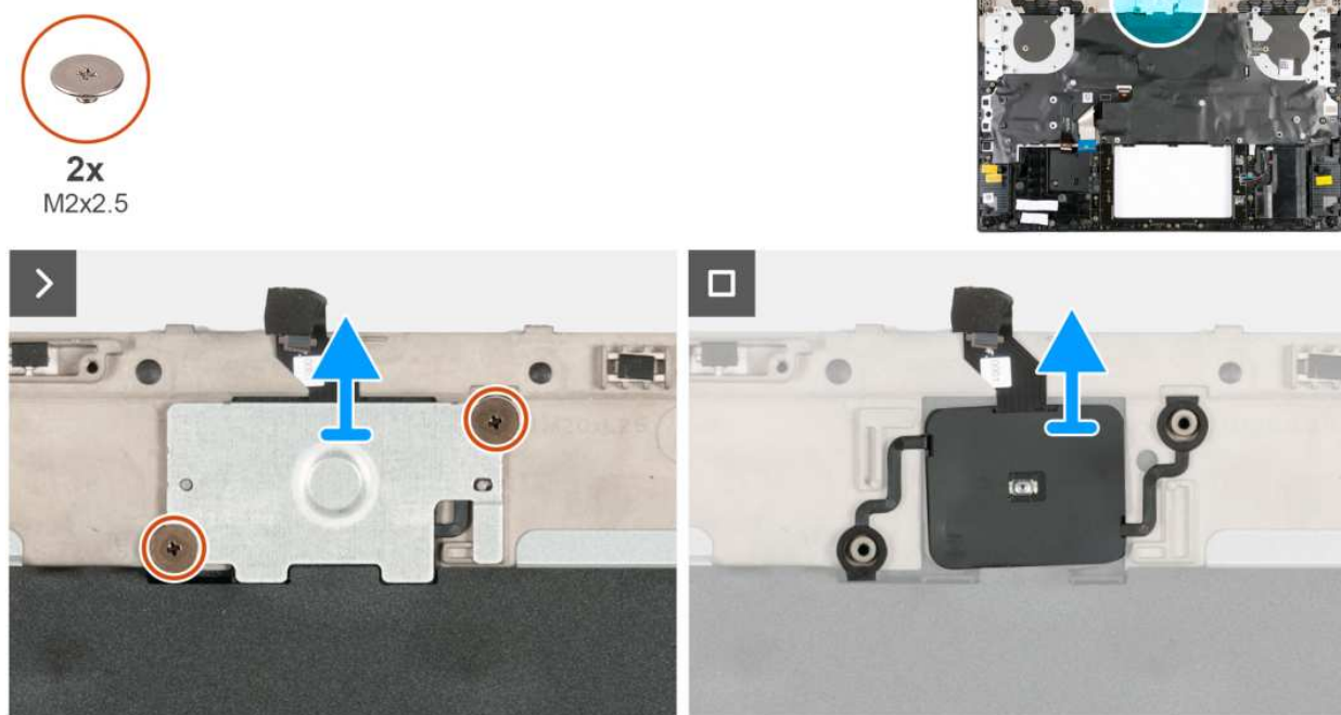
Rysunek 51. Wymontowywanie przycisku zasilania
