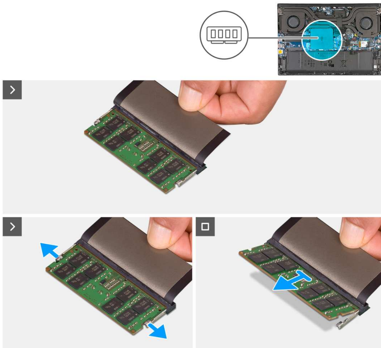
Rysunek 13. Wymontowywanie modułów pamięci
