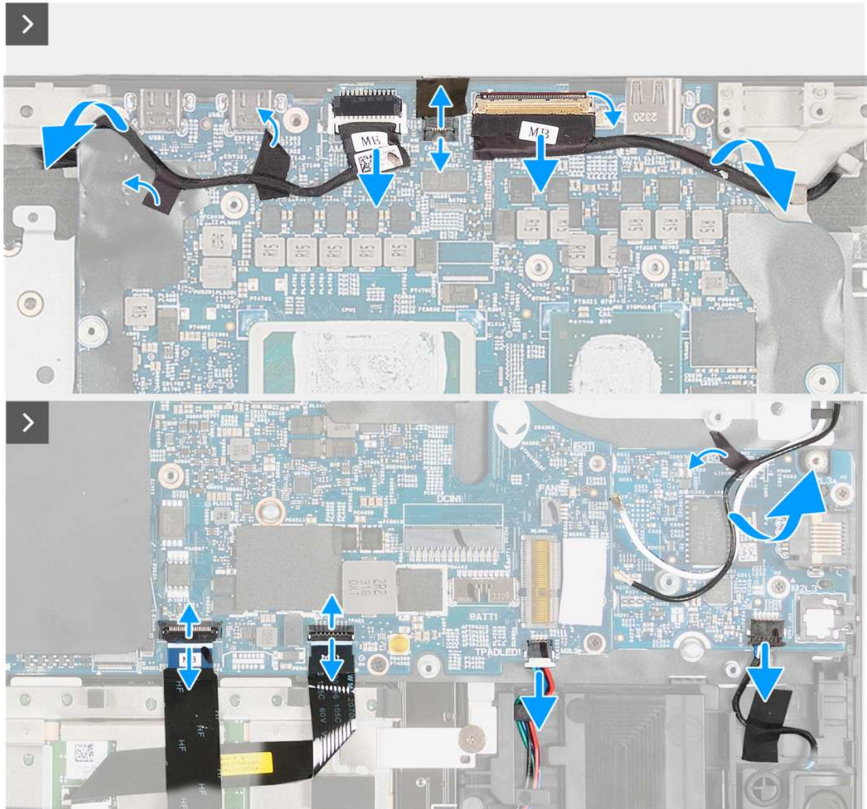
Rysunek 42. Wymontowywanie płyty głównej
