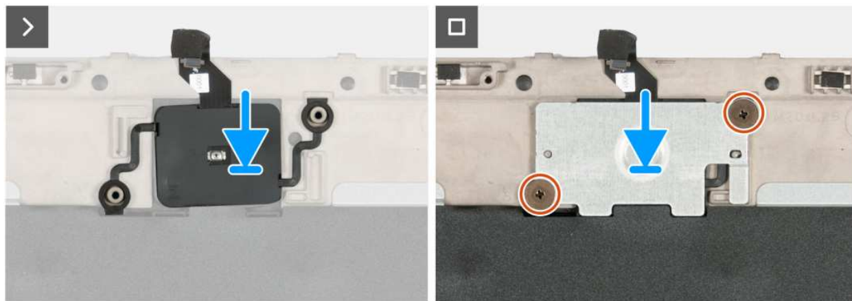
Rysunek 52. Instalowanie przycisku zasilania
