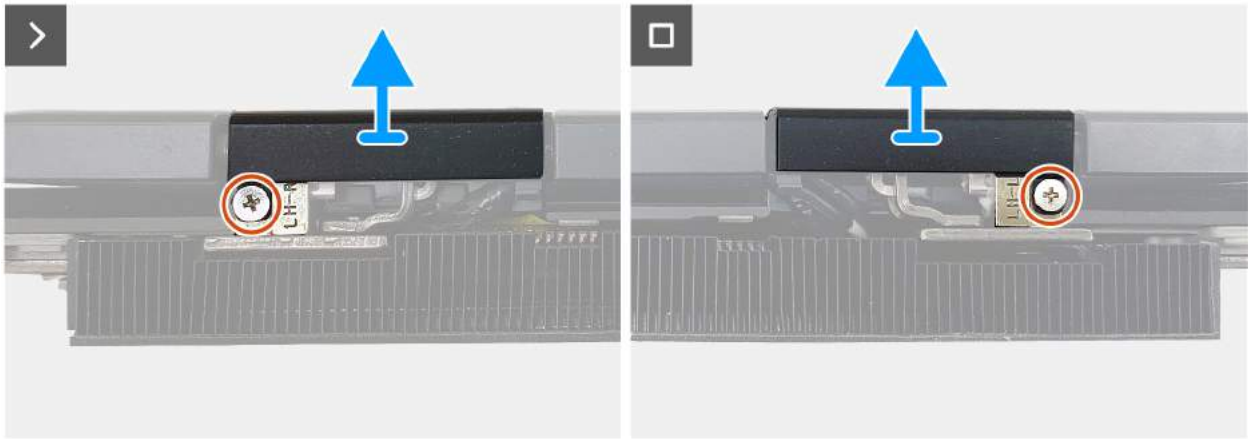
Rysunek 35. Wymontowywanie pokryw zawiasów wyświetlacza
