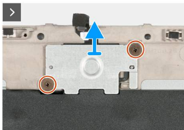
Rysunek 51. Wymontowywanie przycisku zasilania
