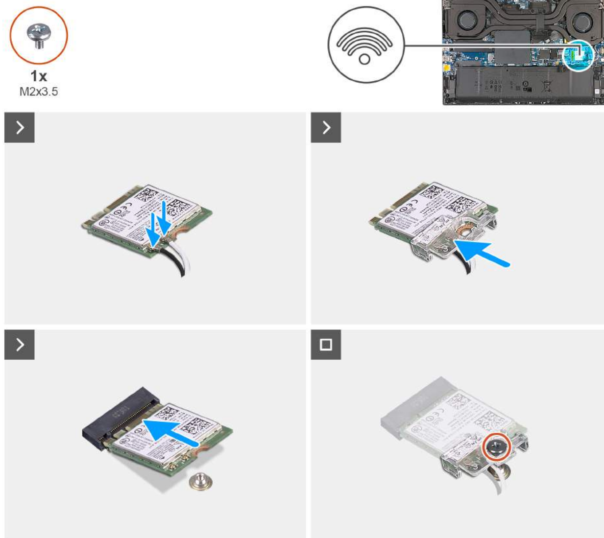
Rysunek 18. Instalowanie karty sieci bezprzewodowej
