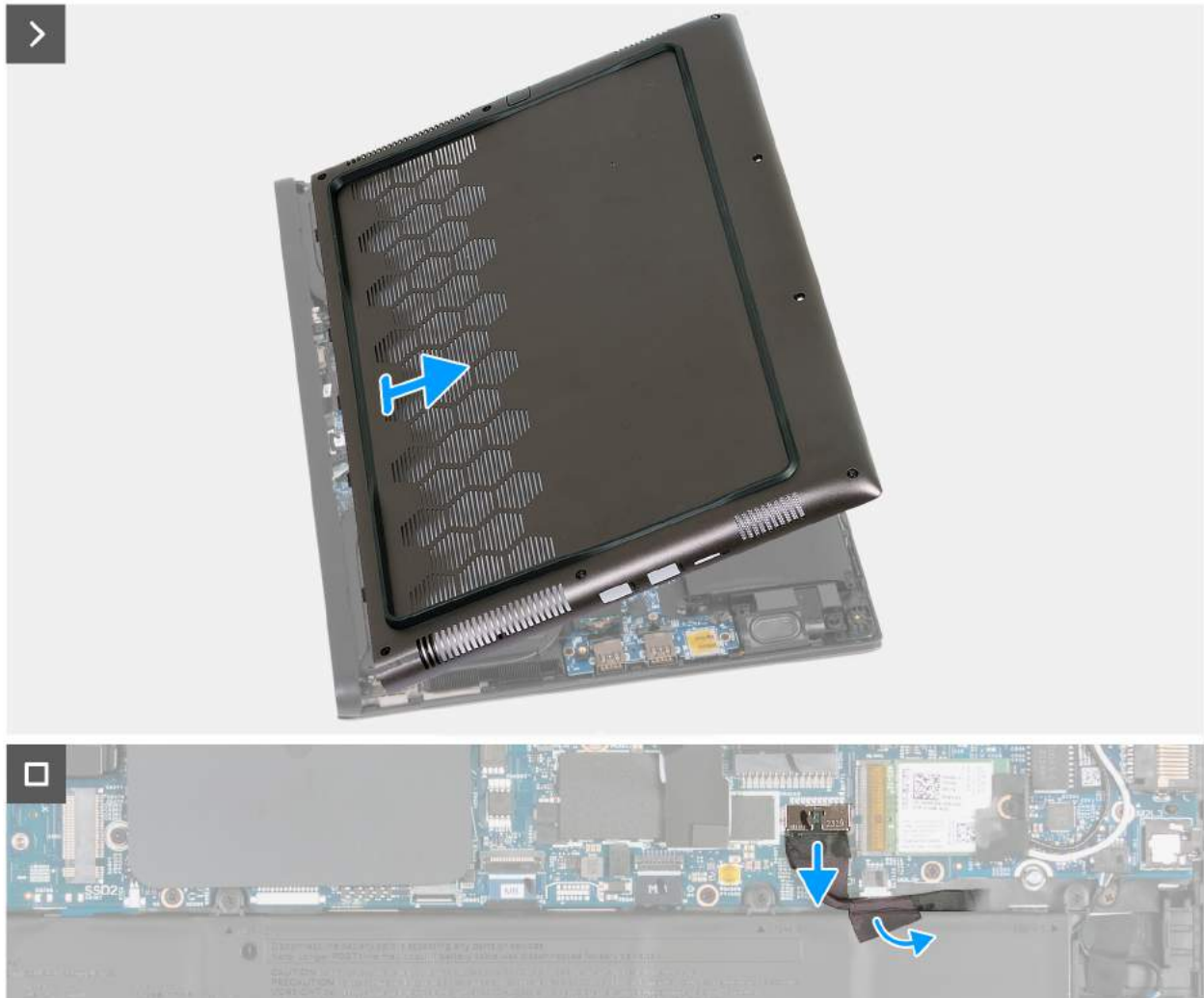
Rysunek 10. Wymontowywanie pokrywy dolnej
