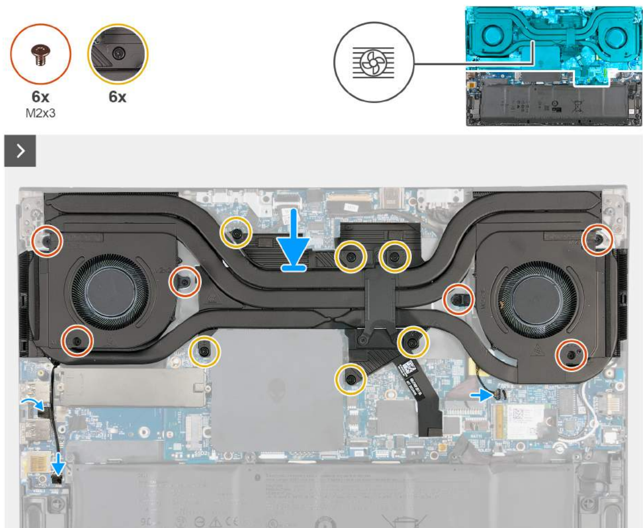
Rysunek 26. Instalowanie zestawu wentylatora i radiatora
