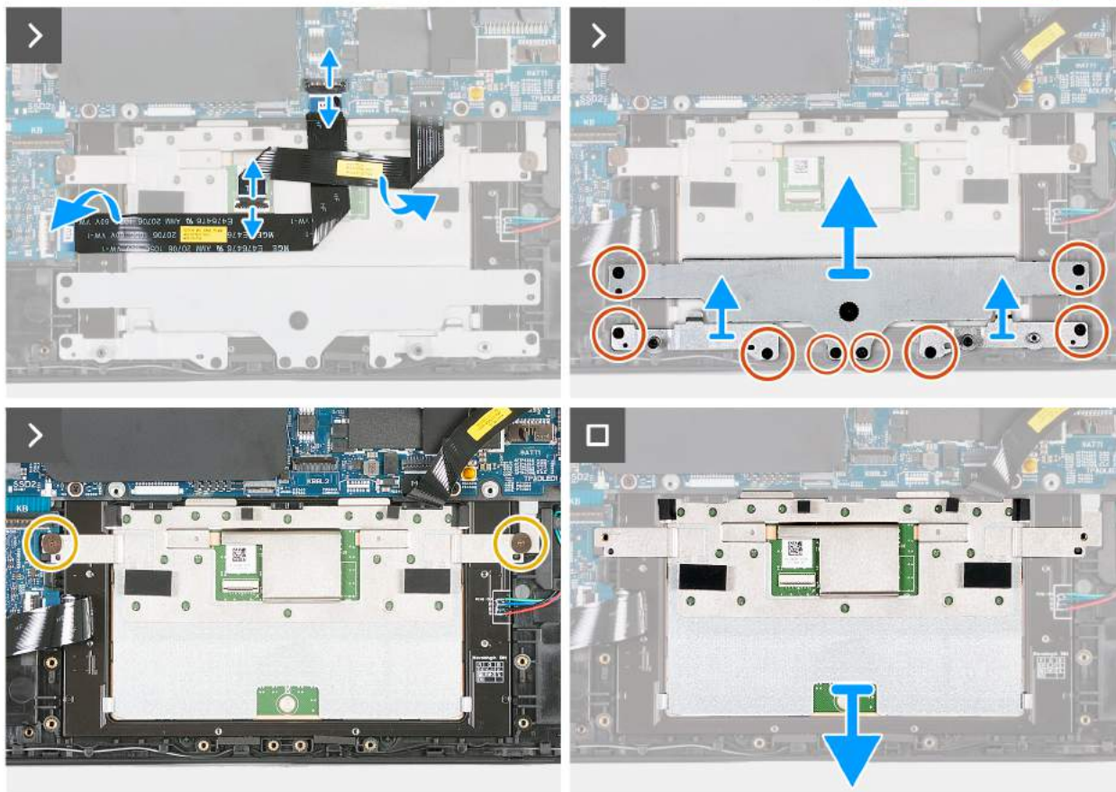
Rysunek 31. Wymontowywanie touchpada
