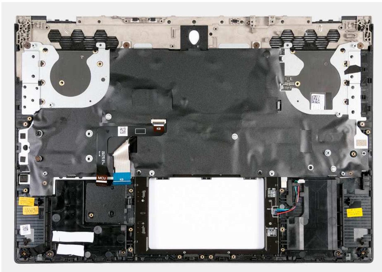
Rysunek 54. Instalowanie zestawu podpórki na nadgarstek i klawiatury
