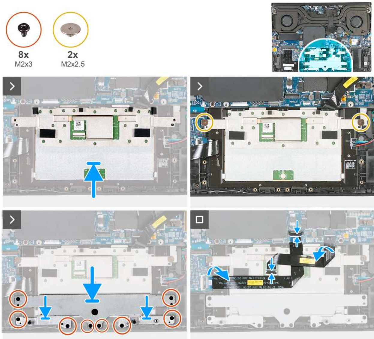
Rysunek 32. Instalowanie touchpada
