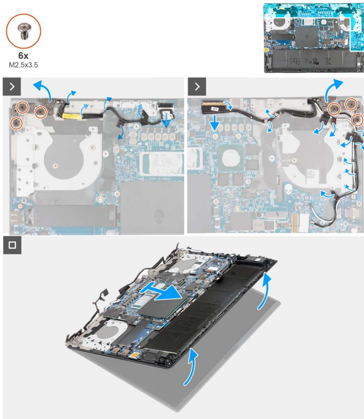
Rysunek 37. Wymontowywanie zestawu wyświetlacza
