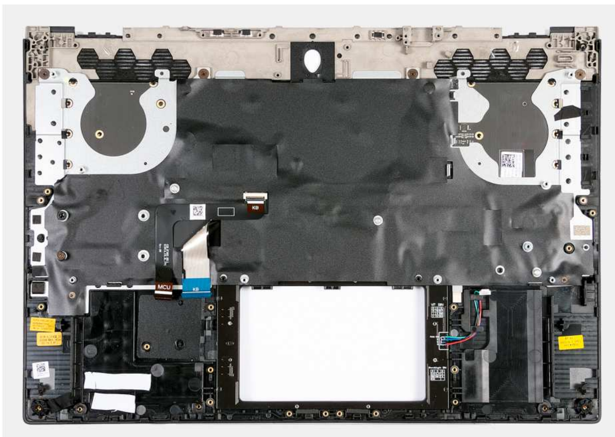
Rysunek 53. Wymontowywanie zestawu podpórki dłoni i klawiatury
