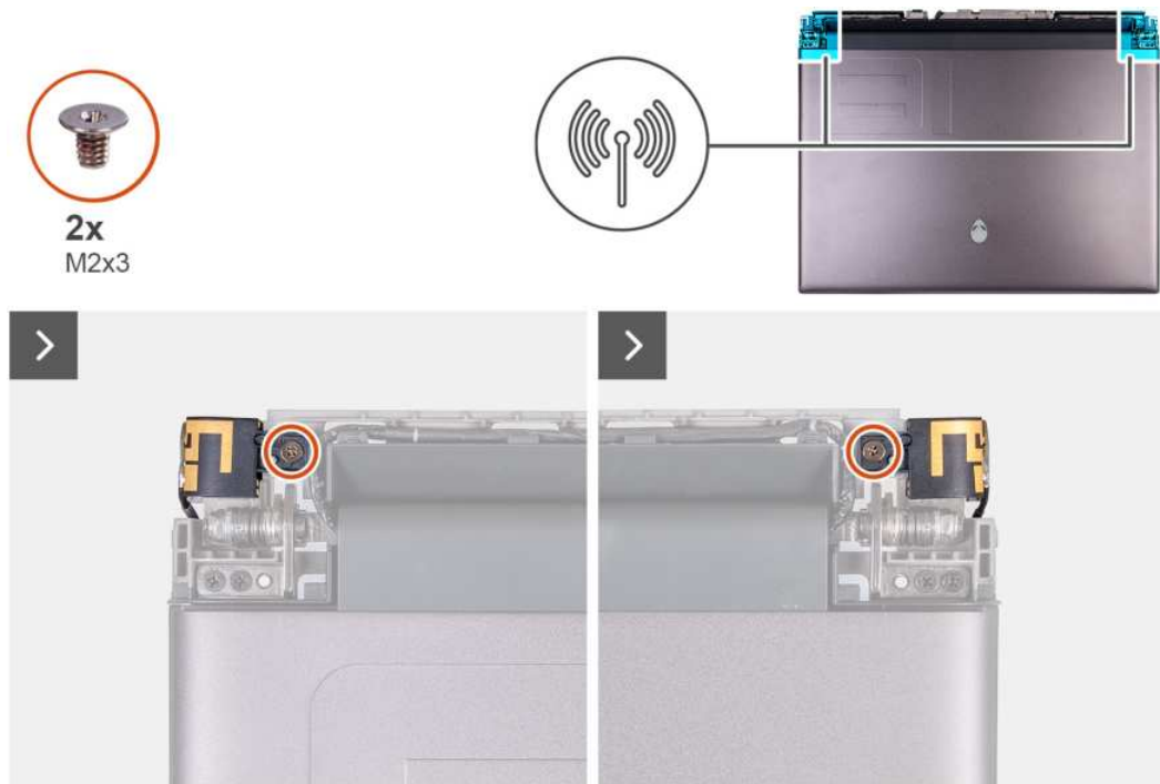
Rysunek 46. Wymontowywanie anteny
