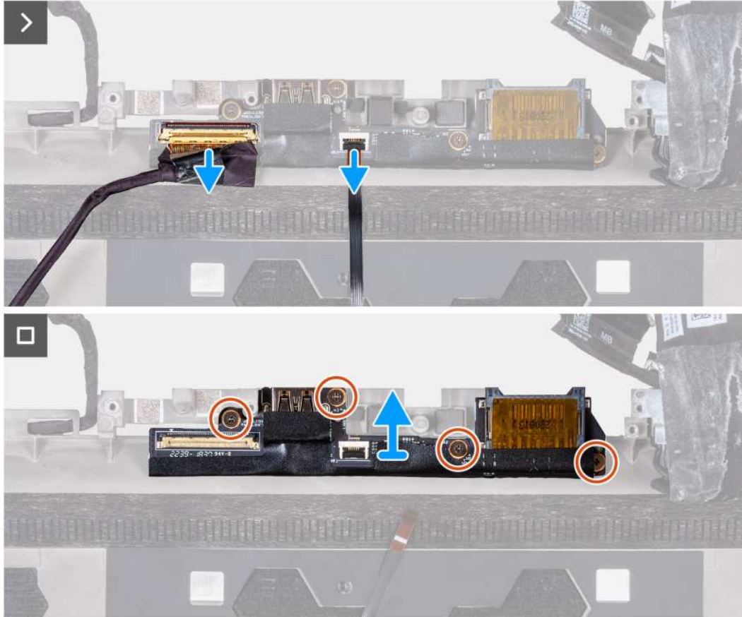
Rysunek 48. Wymontowywanie panelu we/wy
